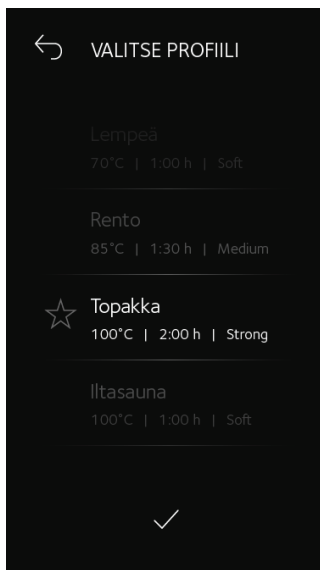
Profiilin valinta
